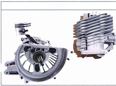
Trykstøbt cylinder med nickel belægning. Stålkrumtap / plejlstang - stempel med 2 stempelringe.
