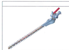
Knivsættet har et klipperområde på 180°. Den justeres trinvis i 12 forskellige positioner. Kan foldes helt ned mod rigrøret under transport.
