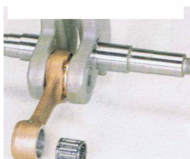
Stål krumtap og 2 stempelringe for reduceret slid og længere levetid.
